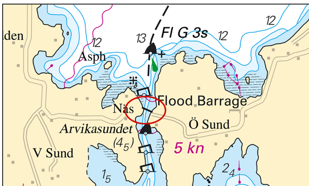
Översvämningsskydd i Arvikasundet
